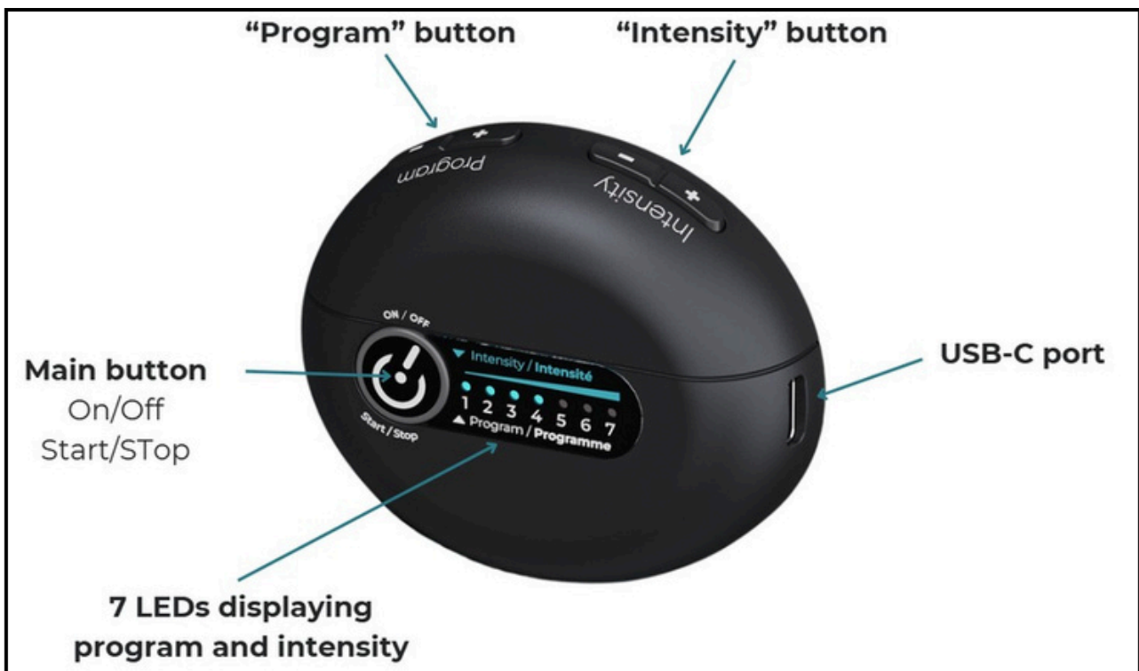
Steuereinheit des neoflo Atemgurtes
